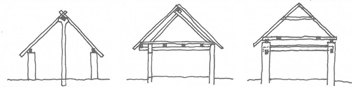
10. ábra - Fedélszék: ágasfás szelemenes; ollóágas; szarufás kötőgerendás, független földemmel (Saját illusztráció)
